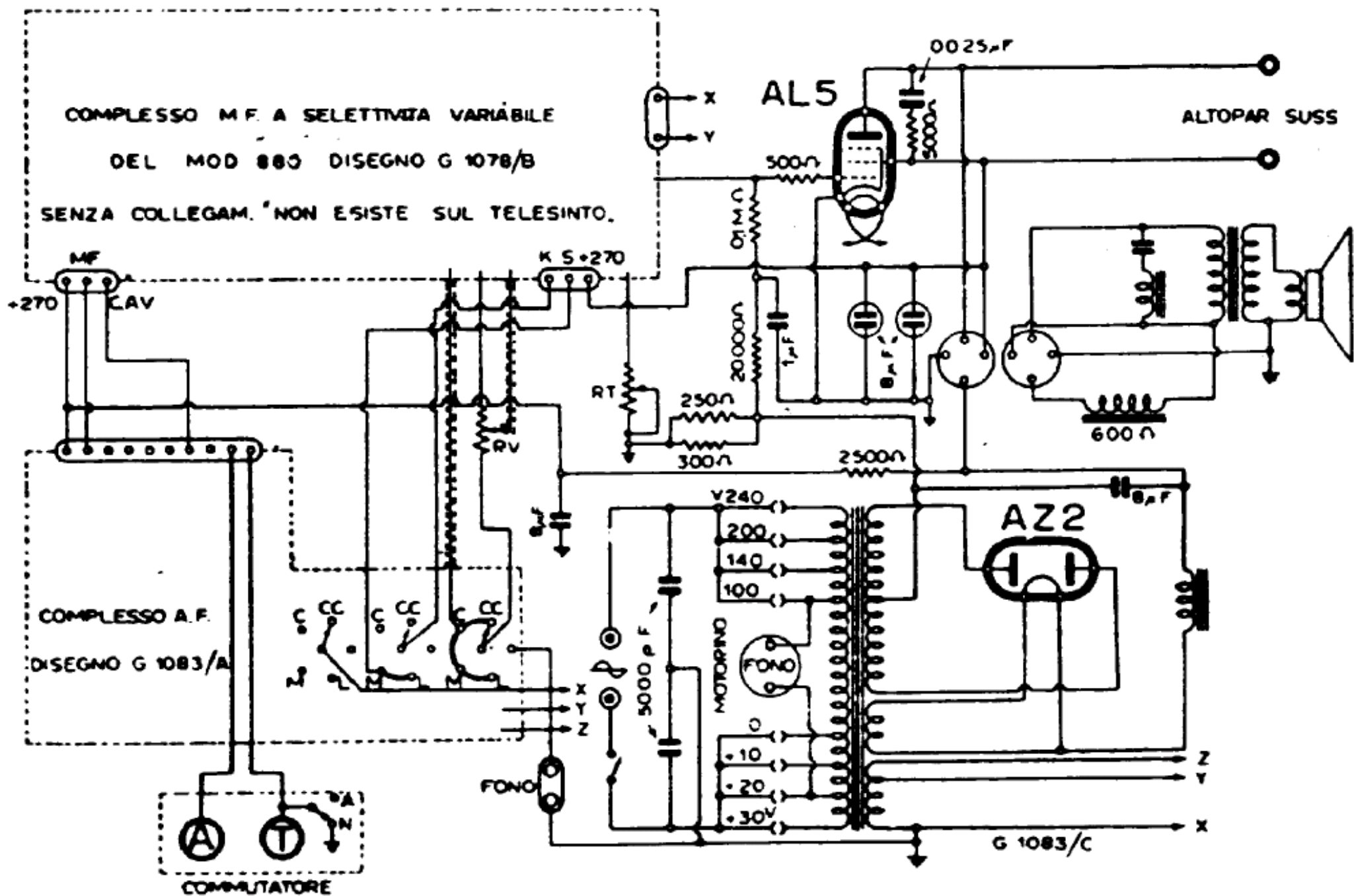
F.I.M.I. - MOD. PHONOLA « 960 » - PARTE BF
